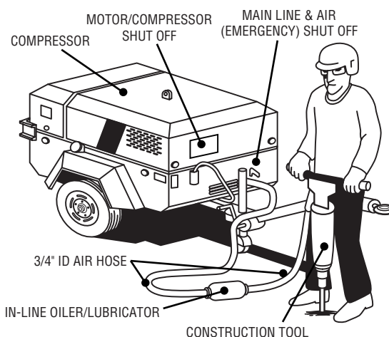
(Dwg. TP2125-1)
